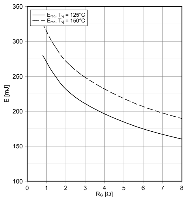
Schaltverluste Diode, Wechselrichter (typisch) switching losses Diode, Inverter (typical)
