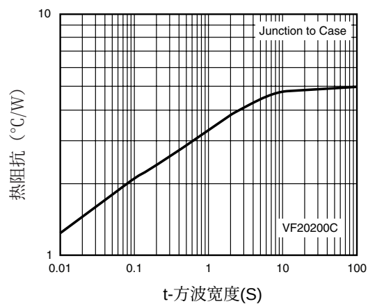
图4 单侧热阻抗
