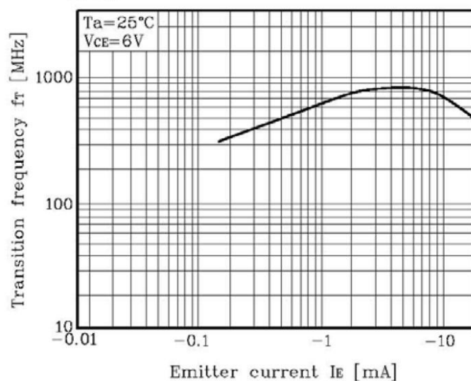
f_T - I_E
