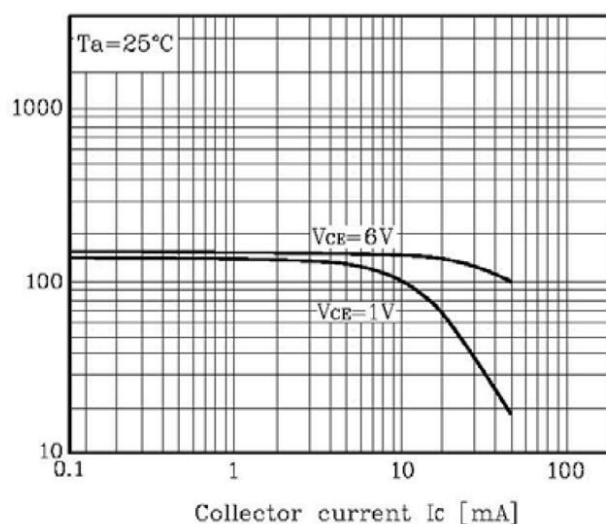
h_{FE} - I_C
