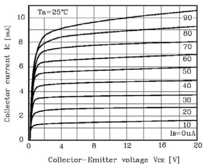
I_C - V_{CE}
