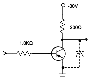
Fig. 1. Turn-On Time
