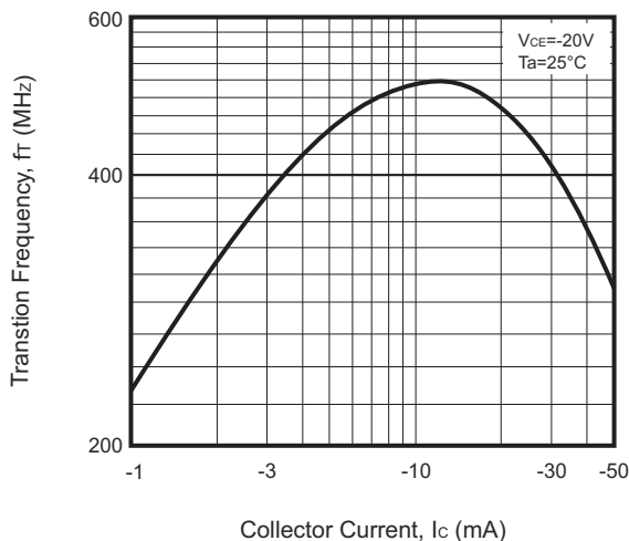
Fig.7 - f_T - I_c
