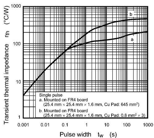
Fig. 7.11 r_{th} - t_w
