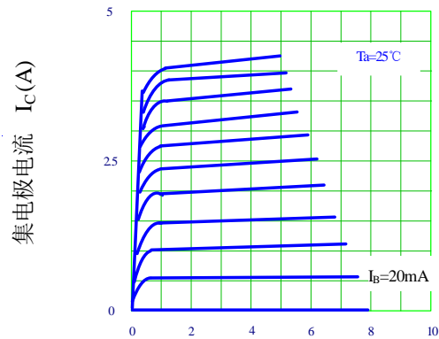
集电极-发射极电压 V_{CE} (V)
