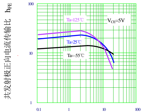
集电极电流 I_C (A)
