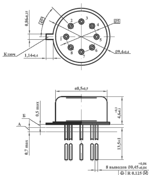
Корпус 3101.8-1, 301.8-2 (дл. выводов 20 \pm 1 \text{ мм} )
