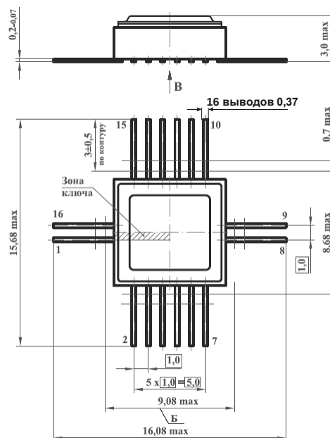
Корпус H04.16-2B
