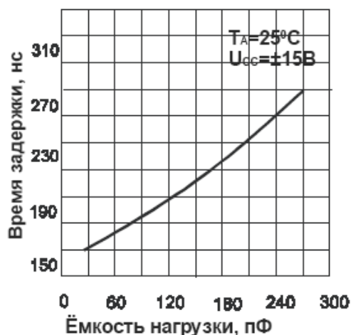
Зависимость времени задержки от ёмкости нагрузки
