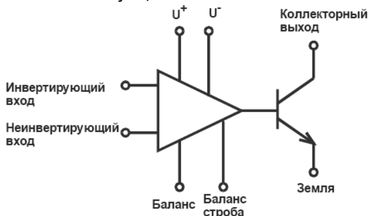
Функциональная схема
