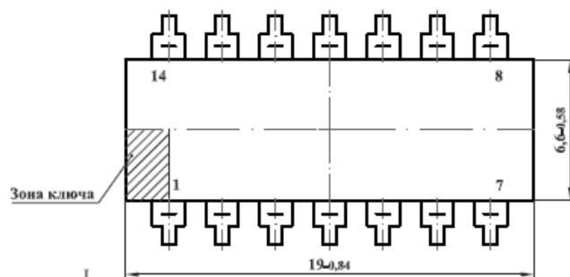
Корпус 201.14-1
