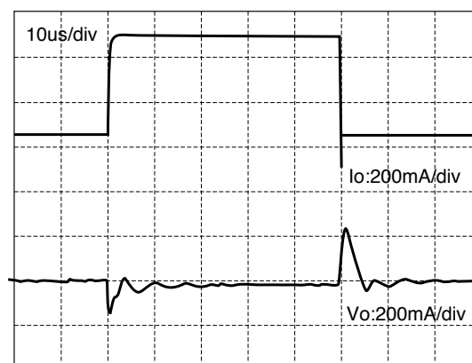
I_o: 50mA \leftrightarrow 500mA
