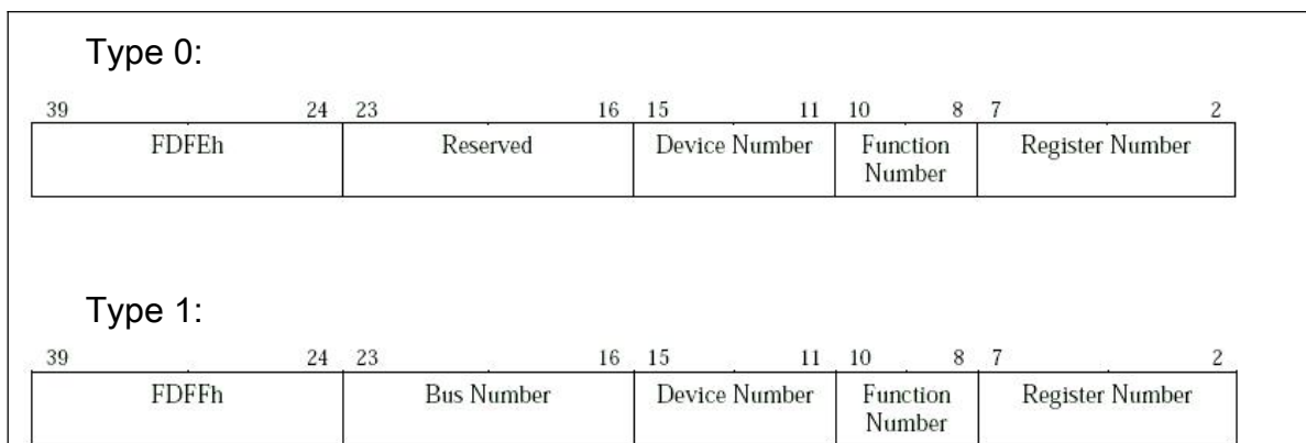
图 10-1 龙芯 3A3000/3B3000 中 HT 协议的配置访问
