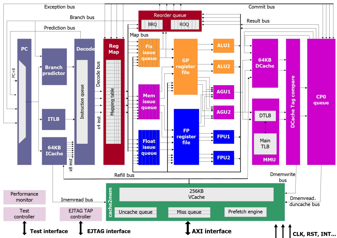
图 3-1 GS464e 结构图
