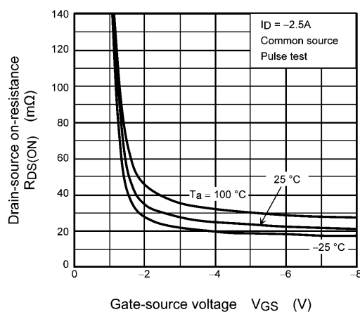
Fig. 7.4 R_{DS(ON)} - V_{GS}
