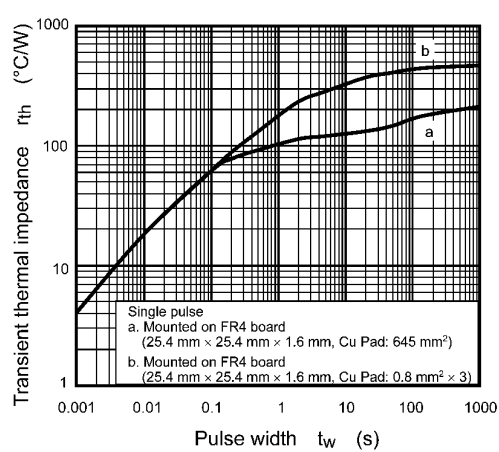
Fig. 7.12 r_{th} - t_w
