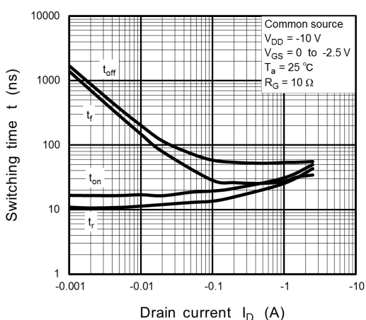
Fig. 7.11 t - I_D
