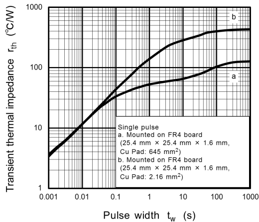
Fig. 8.11 r_{th} - t_w
