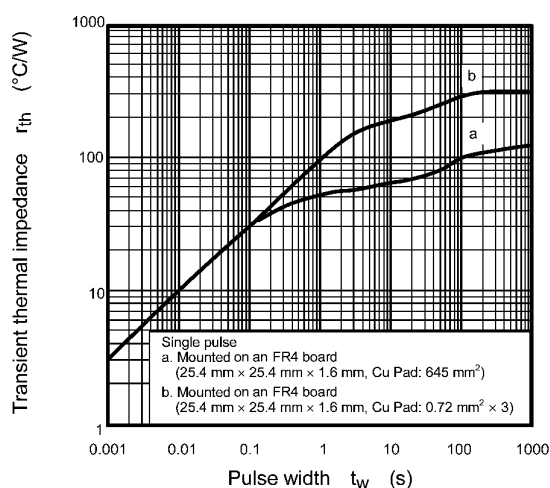
Fig. 7.11 r_{th} - t_w
