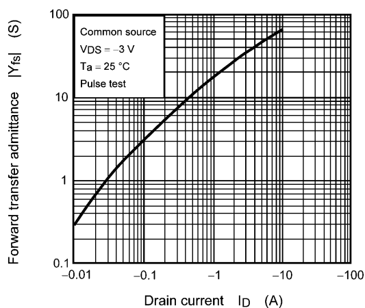
Fig. 8.8 |Y_{fs}| - I_D
