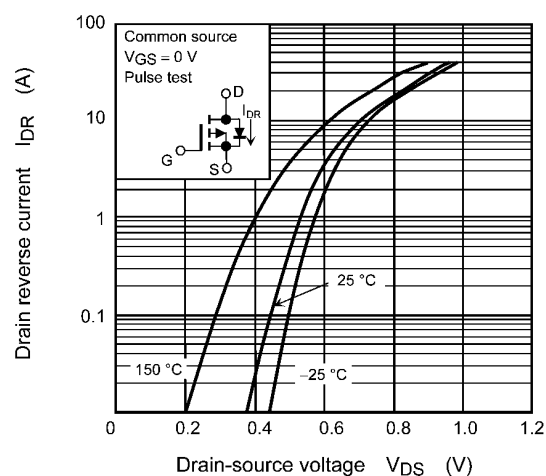
Fig. 8.12 I_{DR} - V_{DS}
