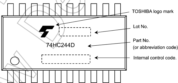
74HC244D
