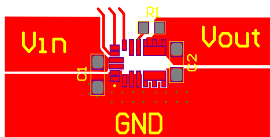
Top Layer
