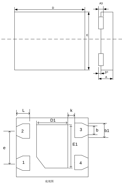
(4)DFN1216-4L 封装
