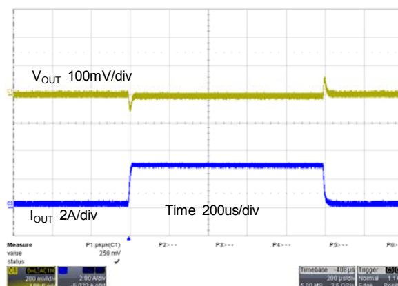
CH3, Fsw=1.5MHz, Iout=100mA~3A, VIN=4.2V
