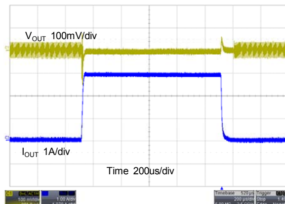
CH1, Fsw=1.5MHz, Iout=100mA~3A, VIN=4.2V
