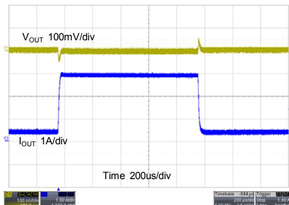
CH1, Fsw=1.5MHz, Iout=500mA~3A, VIN=4.2V
