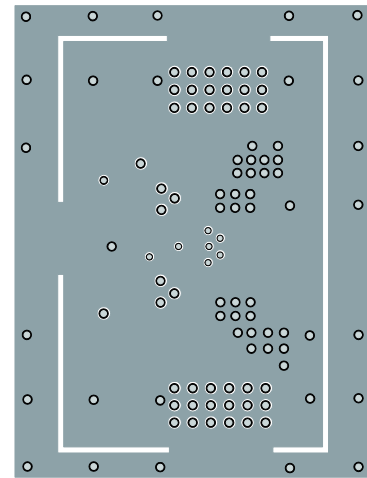
Inner Layer 1
