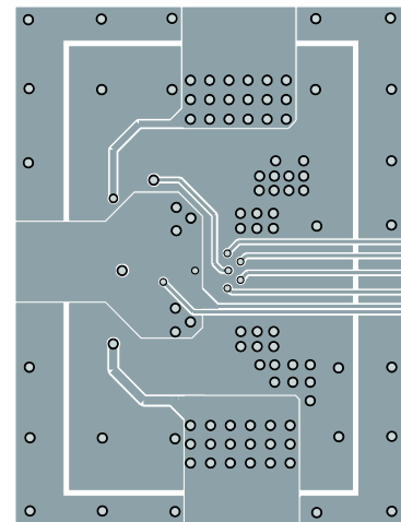
Inner Layer 2
