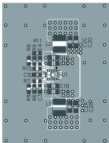
Top Layer
