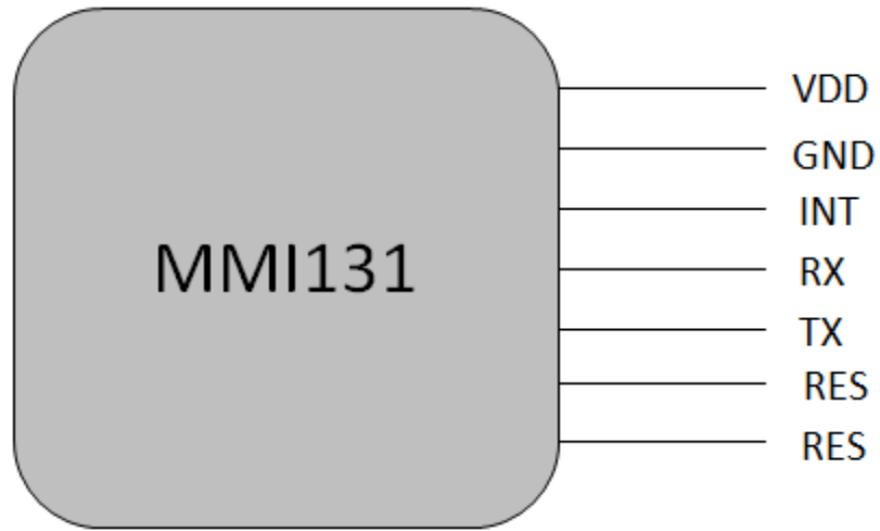
图 1 模块引脚图
