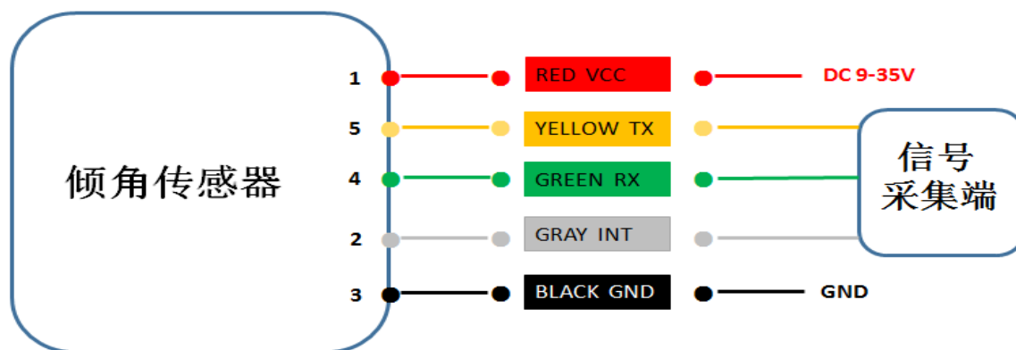
图 3 TTL 连接图
