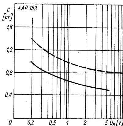
Charakterystyka pojemności diody C = f(U_R)
