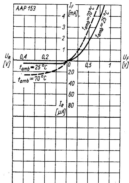
Charakterystyki prądowo-napięciowe
