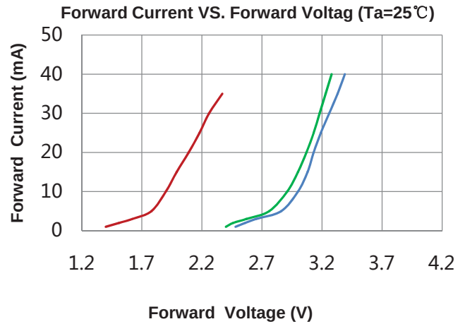
伏安特性曲线
