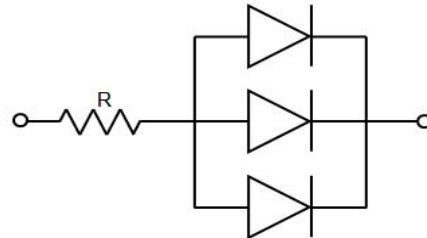
电路模式/ Circuit model B
