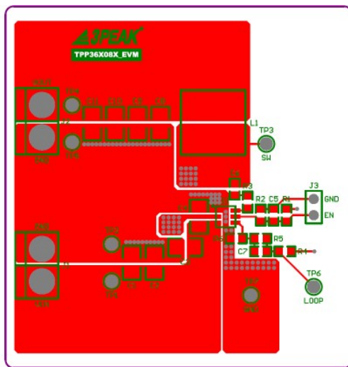
Top Layer
