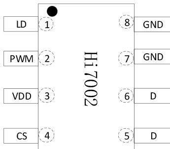
图 5.1 Hi7002 管脚图
