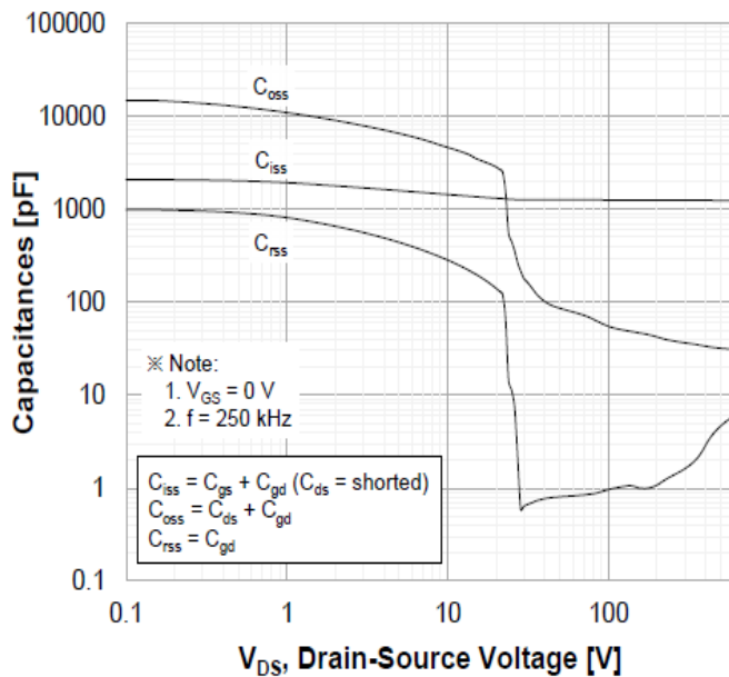
Typ. capacitances
