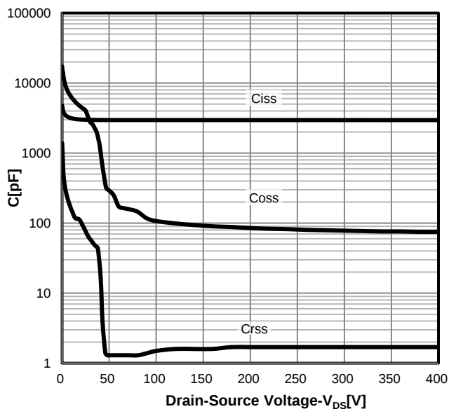
Typ. capacitances
