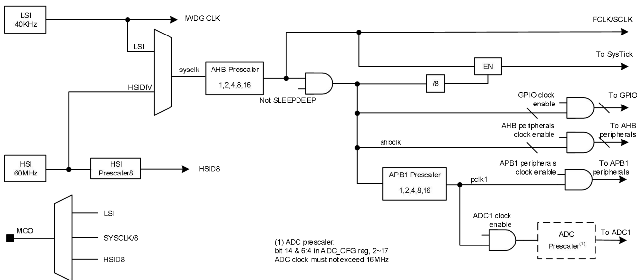
图 3 时钟树
