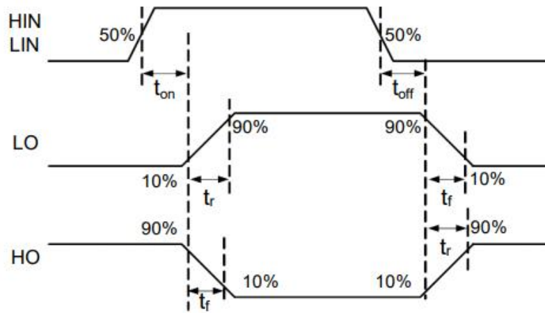
图 26 开关时序
