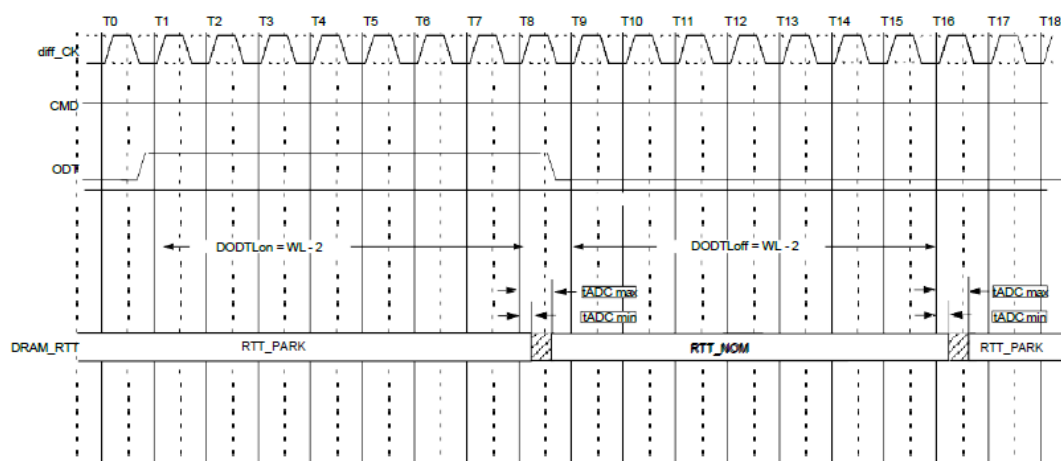
Synchronous ODT Timing Example for CWL=9, AL=0, PL=0; DODTLon=WL-2=7; DODTLoft=WL-2=7
