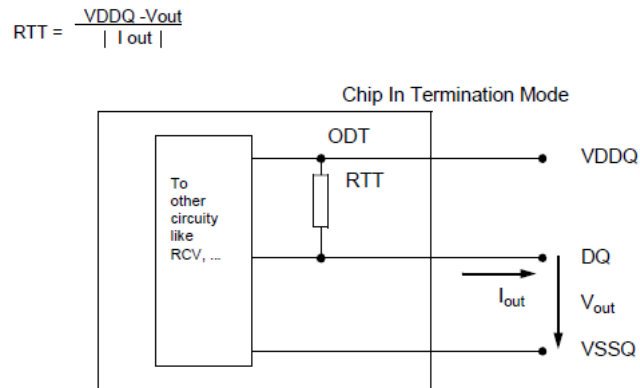
On Die Termination
