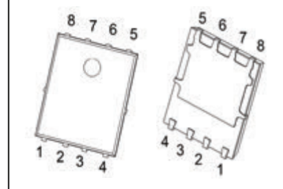
PDFN5x6-8
