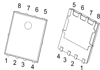
PDFN5x6-8
