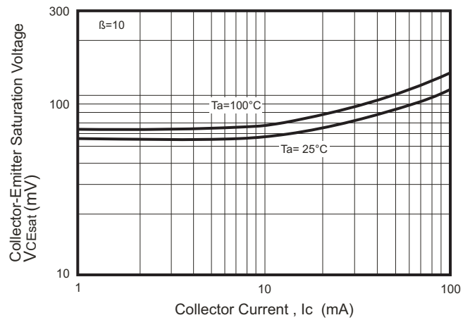
Fig.4 - VCEsat - Ic
