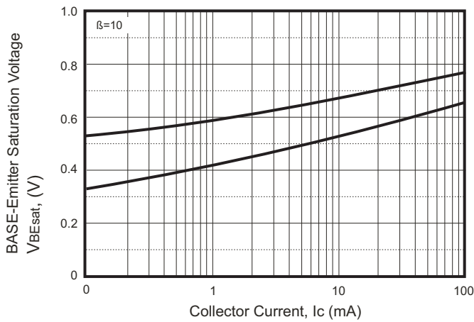
Fig.3 - VBEsat - Ic
