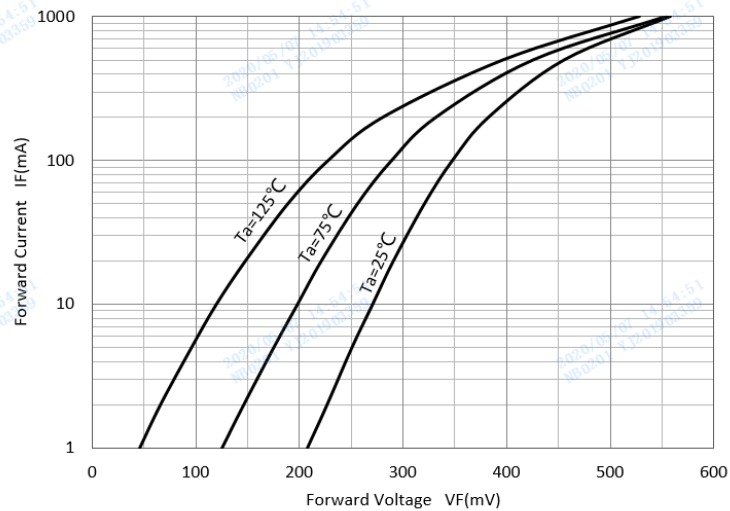
VF-IF
