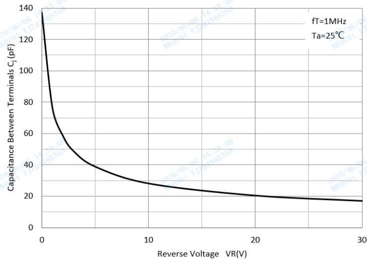
Cj-VR
