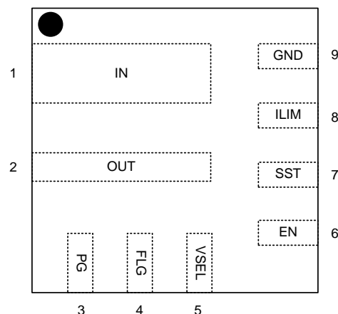
(QFN2x2-9)
