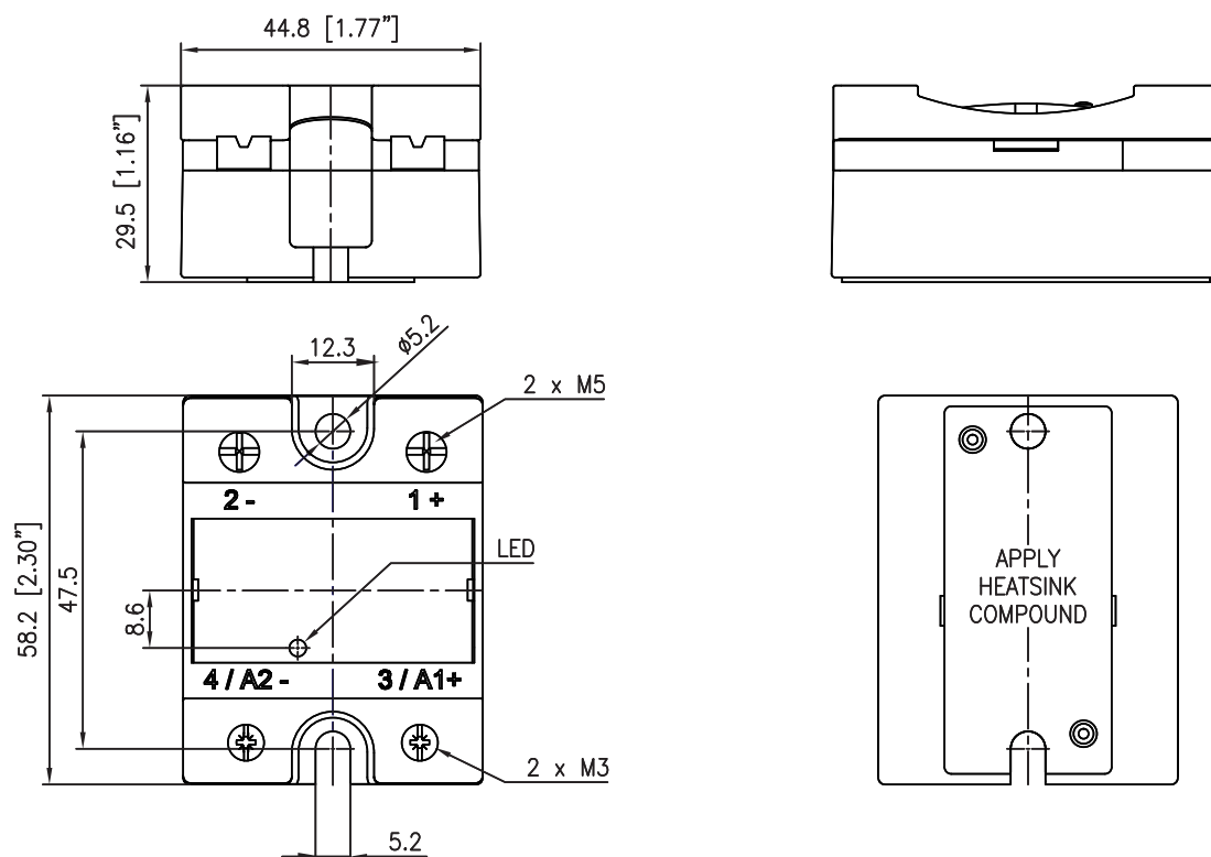
Fig. 1 SHCDC Dimensions
