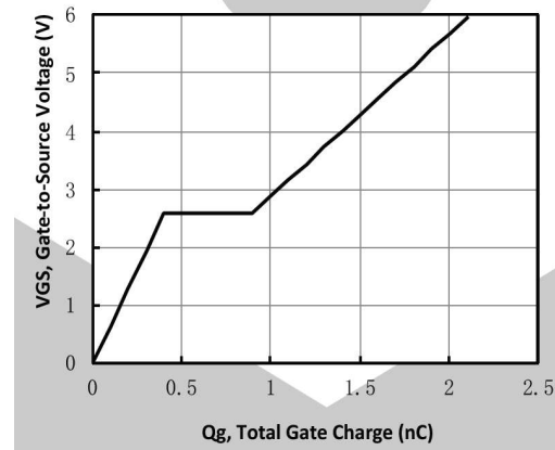
Q_G - V_{GS} curve
