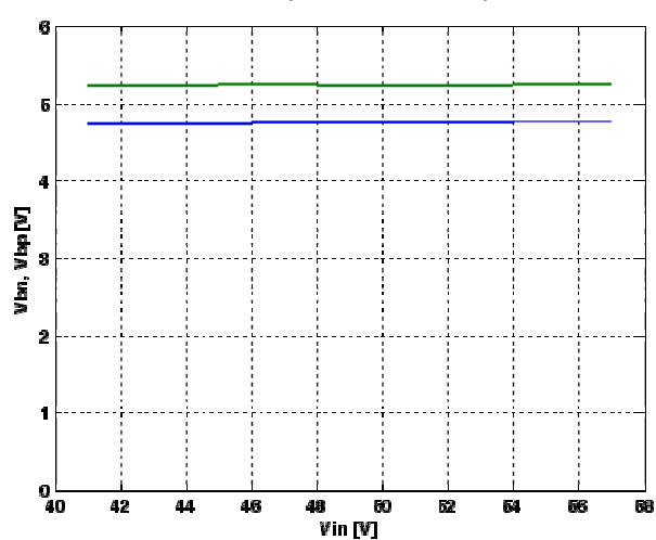
VBN &amp; VBP (VBP wrt VDD480) vs. Vin
