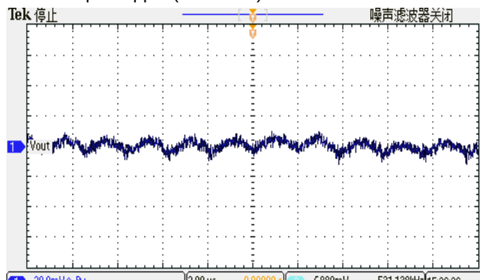
Output Ripple (ILoad=1A)
