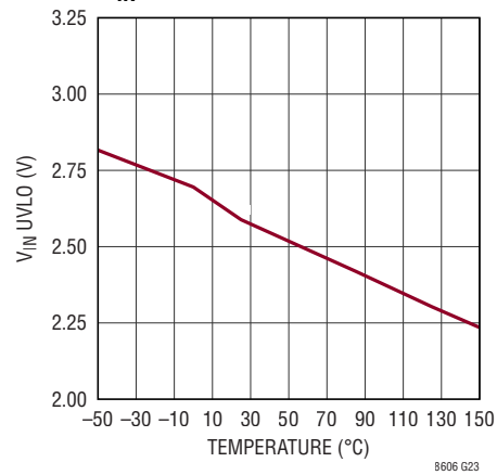
V_{IN} UVLO
