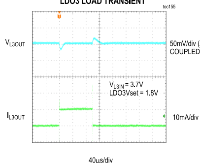
LDO3 LOAD TRANSIENT
