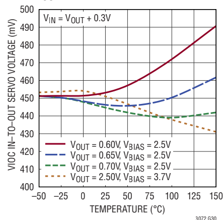
VIOC V_{IN} - V_{OUT} Servo Voltage, I_{OUT} = 10mA
