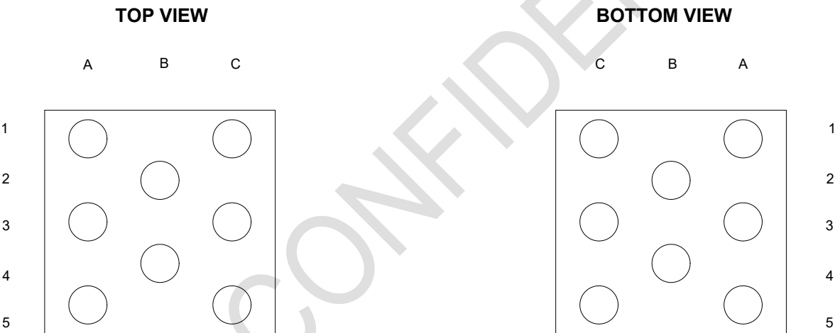
WLCSP8
