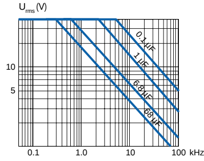
MMK5 63/40
