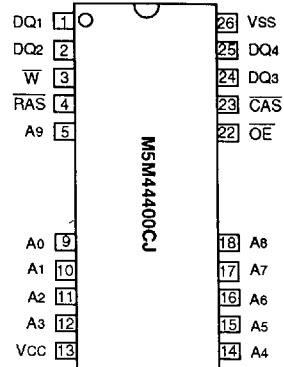
Outline 26P0J(300mil SOJ)
