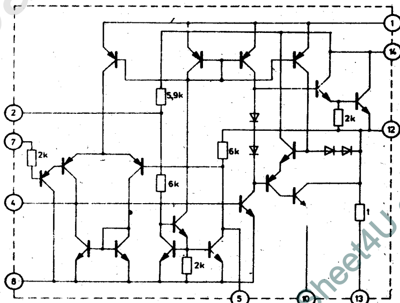
Schema! wewnętrzny
