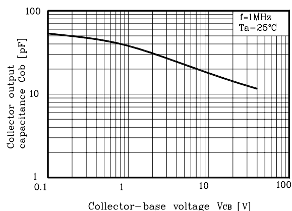
Fig. 7 C_{ob} - V_{CB}
