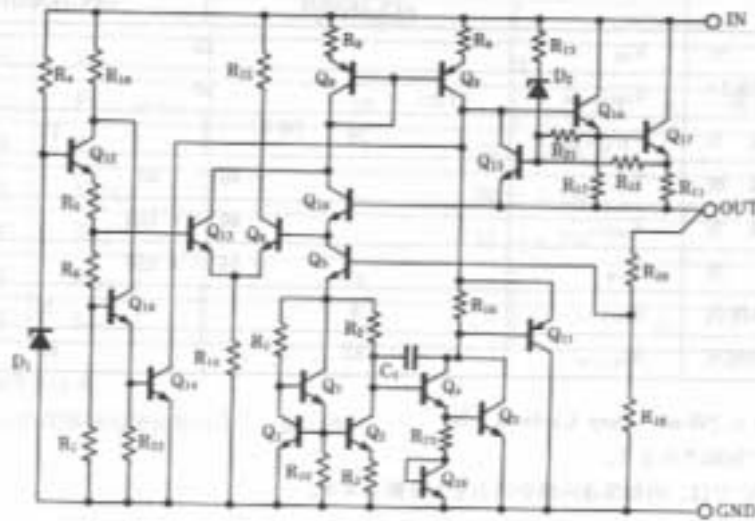
\mu PC14308 ~ 14324, 7808 ~ 7824
