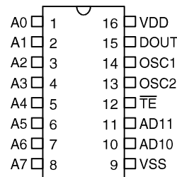
HT12E - 16 SOP
