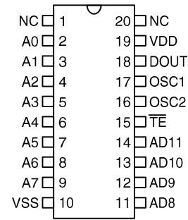
HT12E - 20 SOP
